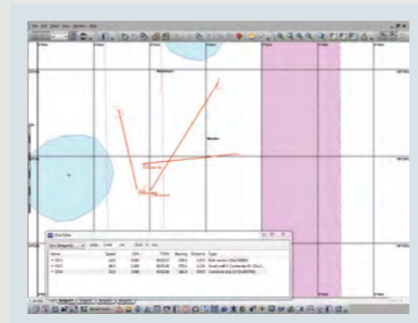
CPA/TCPA
